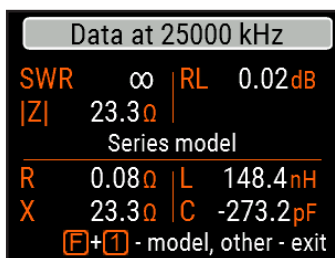
Приклад 2: Невідома індуктивність
